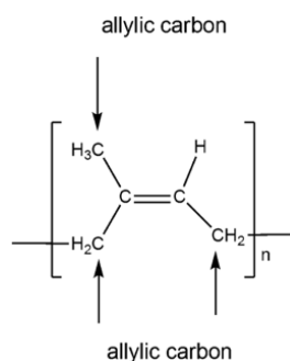
รูปที่ ๑๑ โครงสร้างของยางธรรมชาติที่แสดงหมู่คาร์บอนแอลลิติกและพันธะคู่ (C=C)
