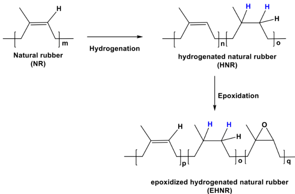
รูปที่ ๘ ปฏิกริยาไฮโดรเจนชันและอีพอกซิเดชันของยางธรรมชาติ
