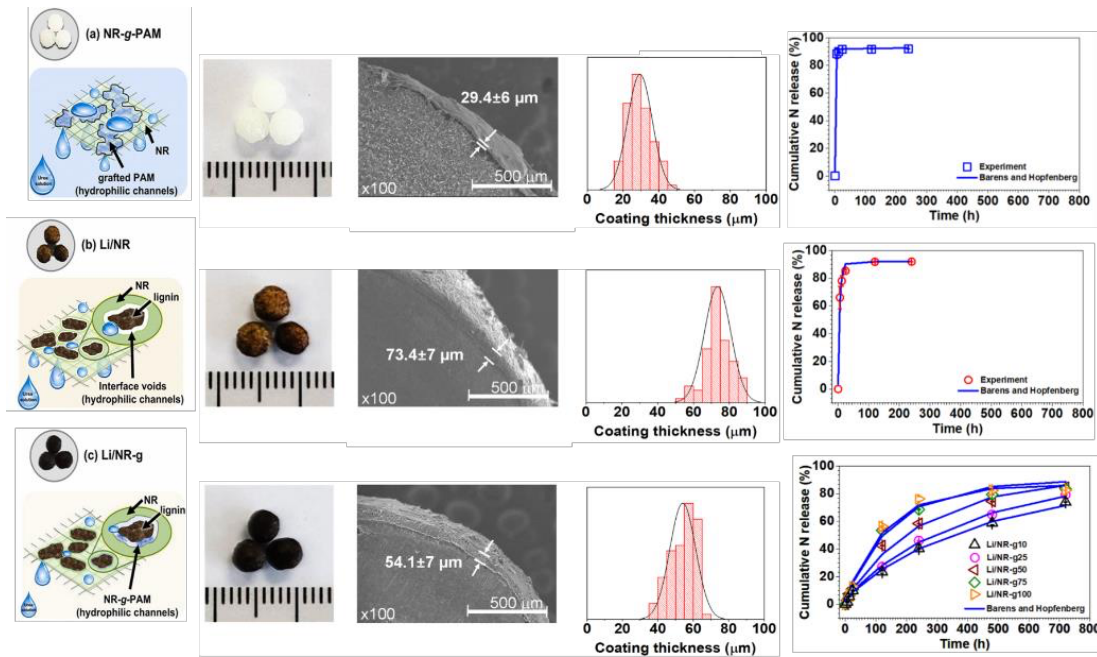
รูปที่ ๔๔ ภาพร่าง ภาพถ่ายเม็ดปุ๋ย ภาพถ่าย SEM (ตัดขวาง) แสดงความหนาของชั้นเคลือบ และกราฟแสดงรูปแบบการปลดปล่อยไนโตรเจนของเม็ดปุ๋ยยูเรียเคลือบด้วยคอมพอลิเมอร์ชีวภาพลิกนินผสมยางธรรมชาติที่มีการเติมยางธรรมชาติกราฟต์พอลิอะคริลาไมด์ (Boonying et al., 2023)
